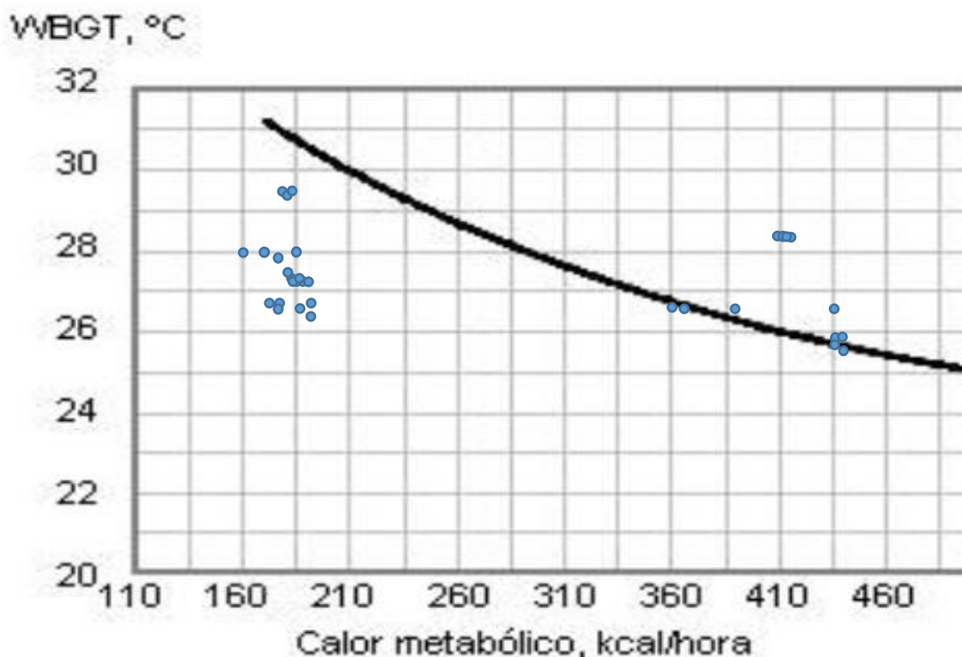
Gráfico 1. Relación entre el índice de calor WBGT y el calor metabólico para la identificación de riesgo de sufrir estrés térmico, acorde con la norma NTP 322 33
